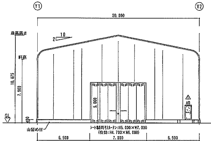
X1通り側立面図 S=1:200
