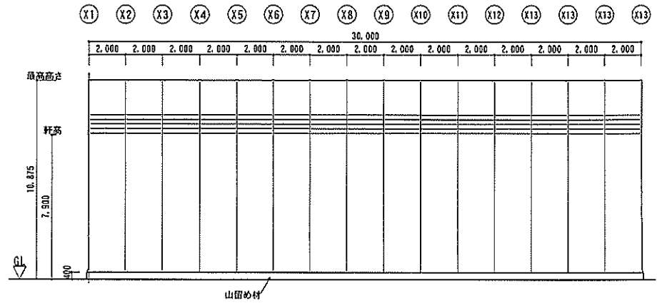
Y1 (Y2)通り側立面図 S=1:200
