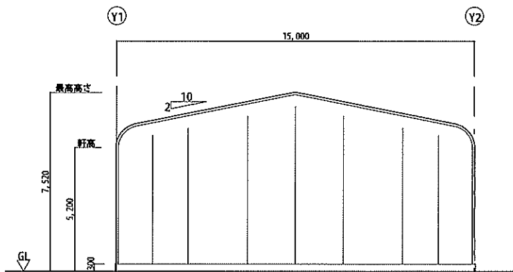
X1通り側 立面図 S=1:150
