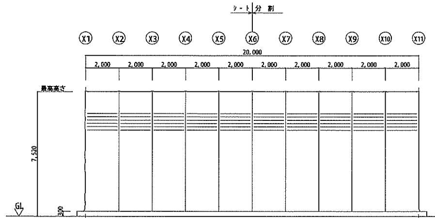
Y1(Y2)通り側 立面図 S=1:150
