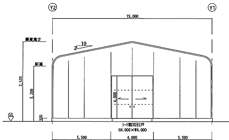
X1通り側 立面図 S=1:150
